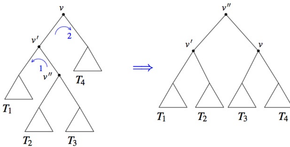
Abbildung 5.6: Doppellinksrotation DRotLinks(v, v', v'') .
