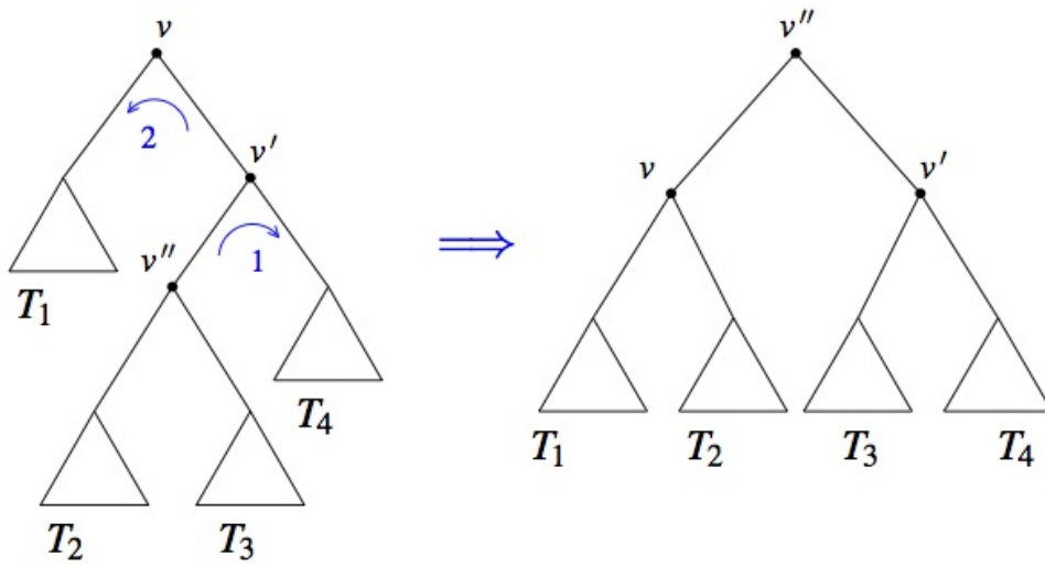
Abbildung 5.6: Doppellinksrotation DRotLinks(v, v', v'') .
